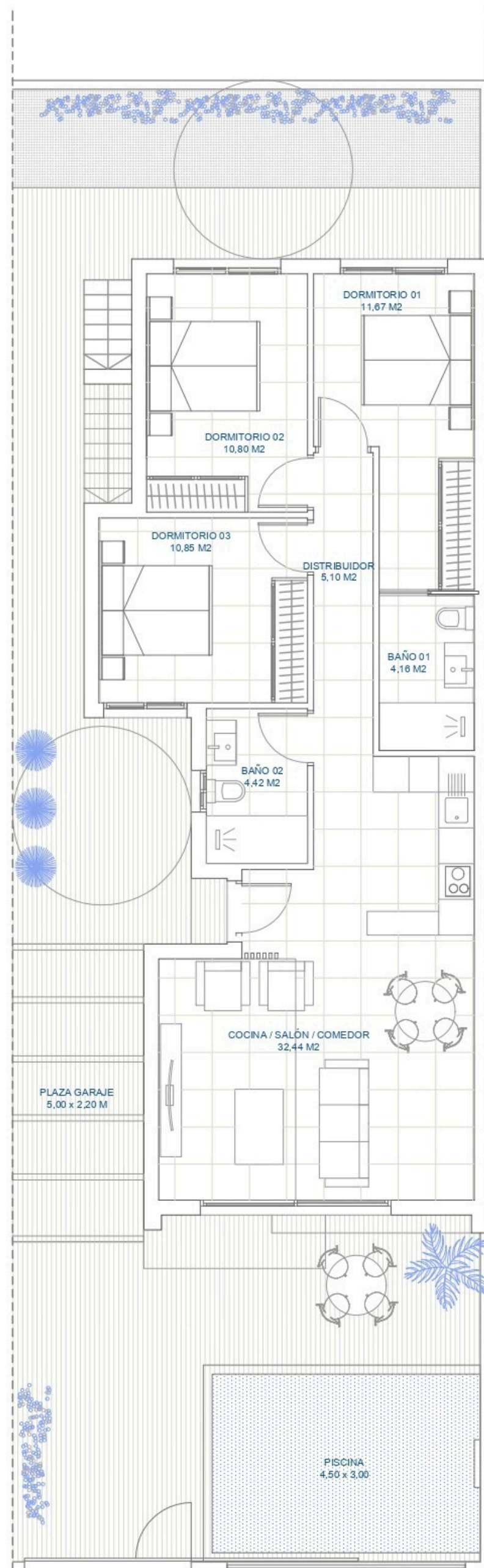
PLANTA BAJA
