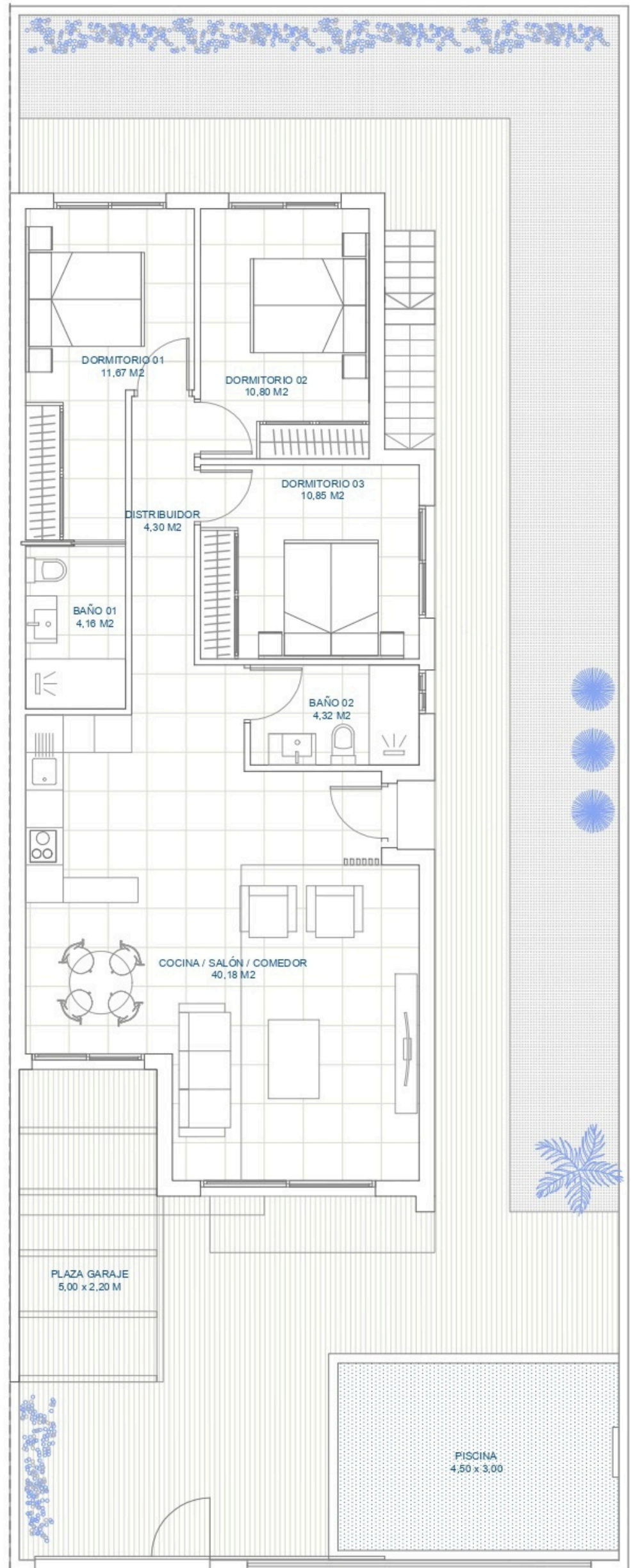
PLANTA BAJA
